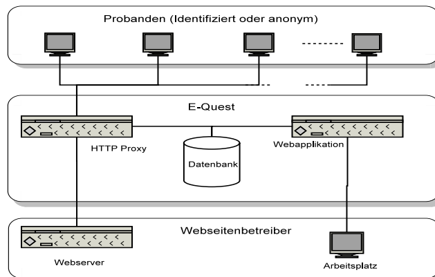
Abbildung 3: Architektur des Evaluations-Tools
